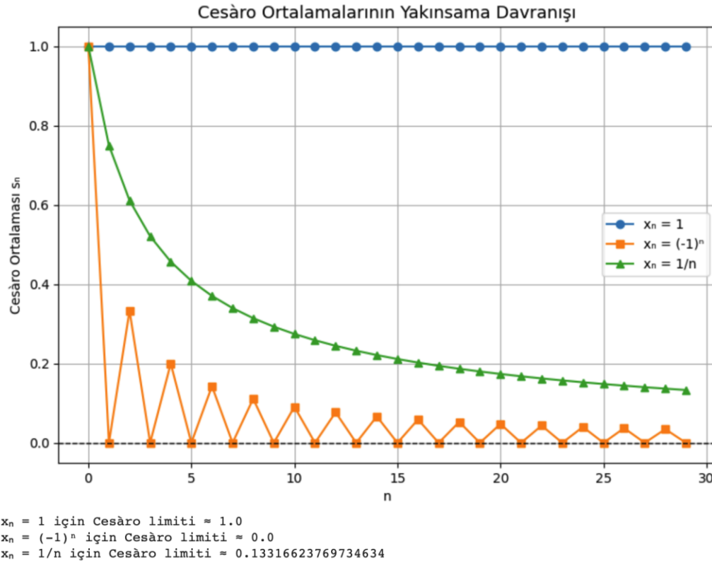
Görsel 2. Cesàro ortalamalarının yakınsama davranışı
