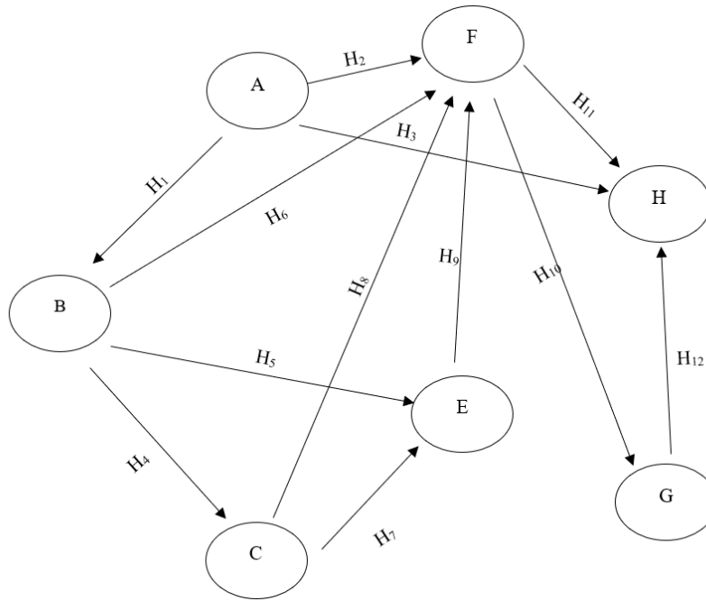
Şekil 1: Araştırma Modeli
