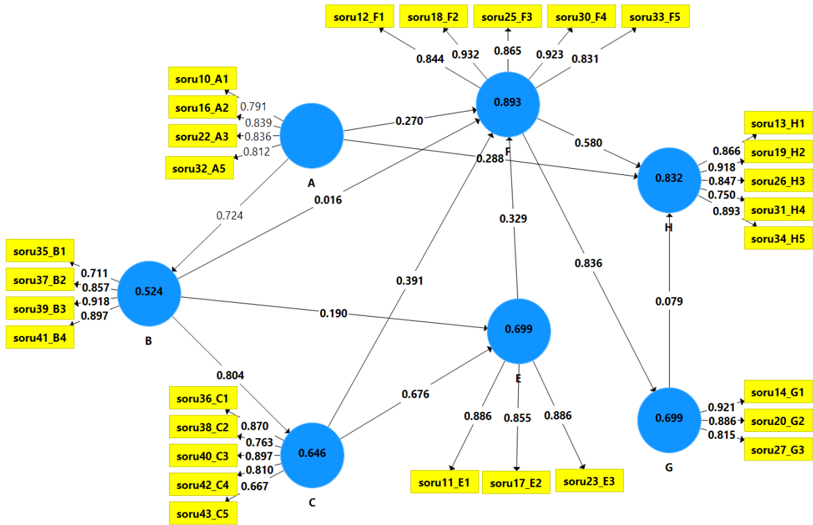
Şekil 2: KEKK-YEM diyagramı
